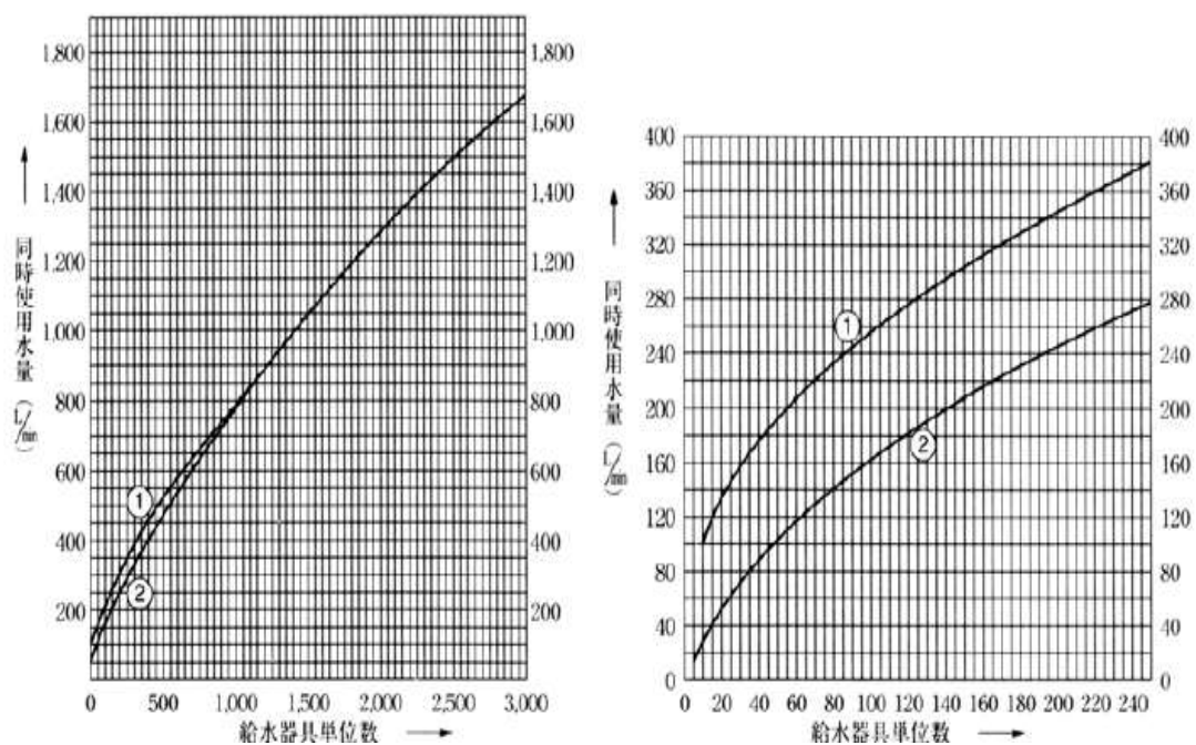
【図 4.3.1 給水用具給水負荷単位による同時使用水量図】
