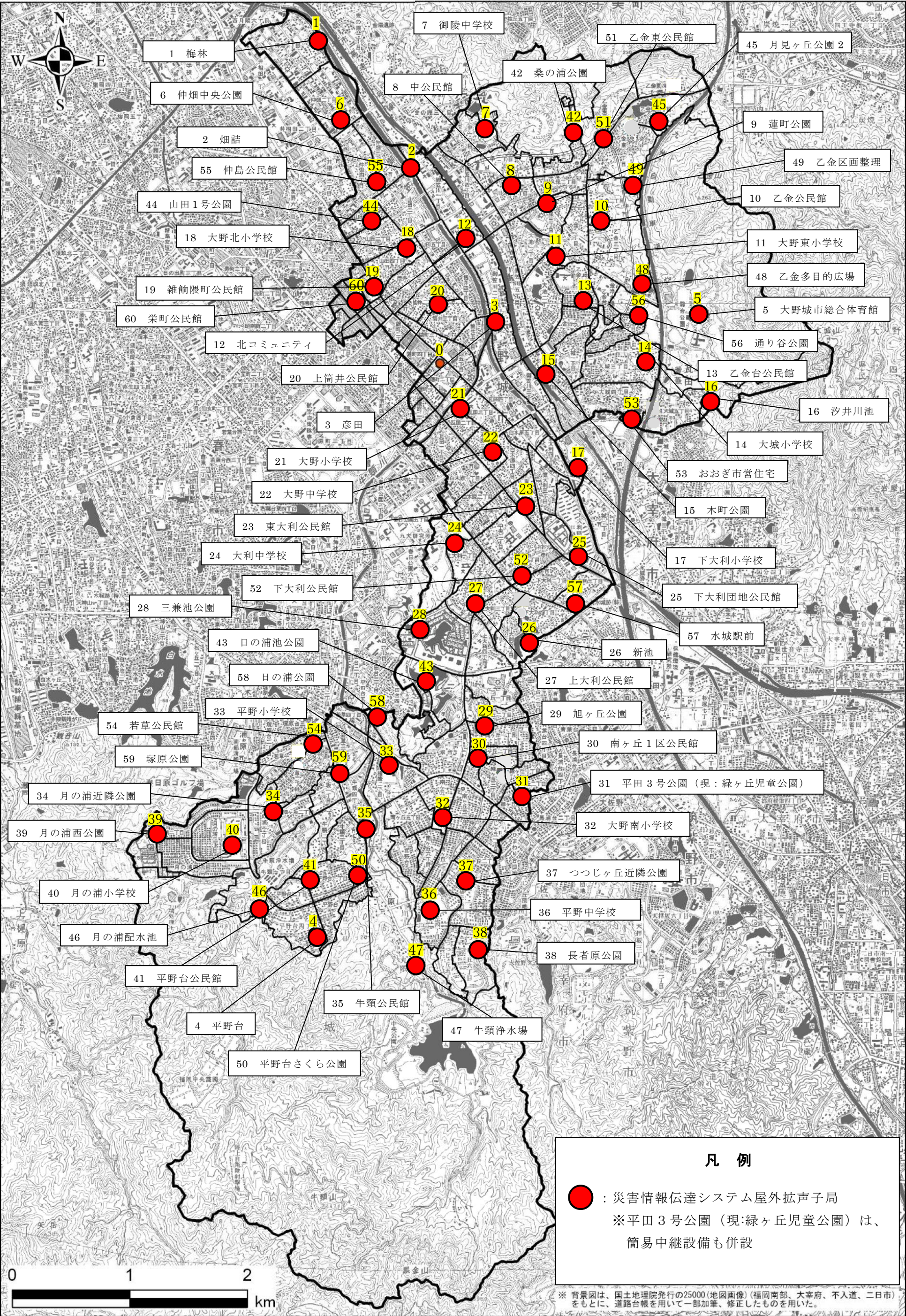
■災害情報伝達システム 屋外拡声子局設備 位置図
